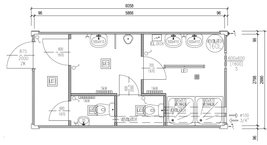
SANITÄRCONTAINER S11
