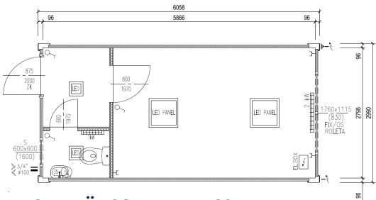
SANITÄRCONTAINER S3
