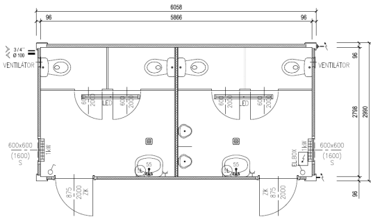
SANITÄRCONTAINER S7
