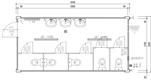
SANITÄRCONTAINER S6
