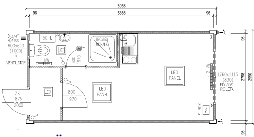
SANITÄRCONTAINER S4
