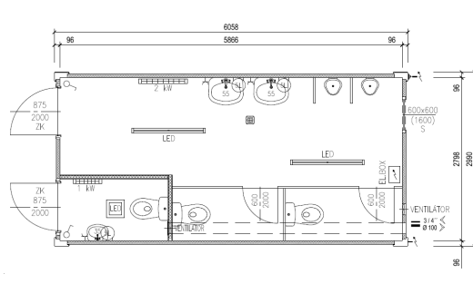
SANITÄRCONTAINER S8
