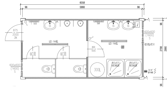
SANITÄRCONTAINER S10
